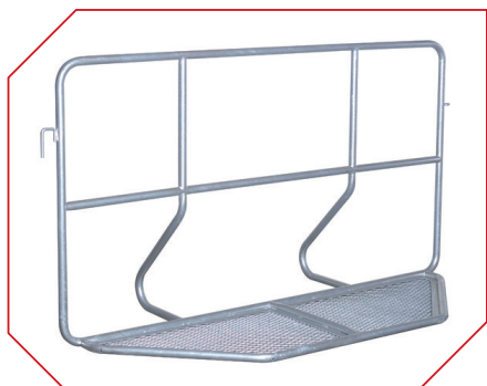
Polizeigitter Starr Abmessung: L 2,088 mm x 1,200 mm Vollfeuerverzinkt
