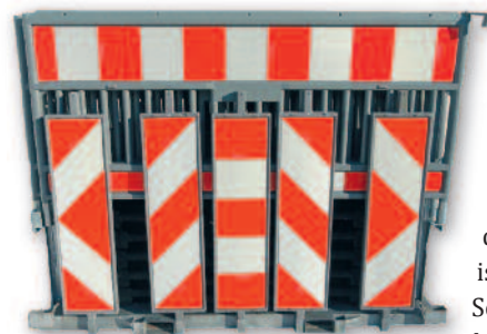
Auf der KP 22 M LL können längs und quer auf einmal transportiert oder verladen werden: 20 Absperrschranken, 28 Multi-Fußplatten K 1 und 10 Leitbaken. In einer integrierten Box können zudem noch Ersatz-Batterien und Kleinteile transportiert werden.
